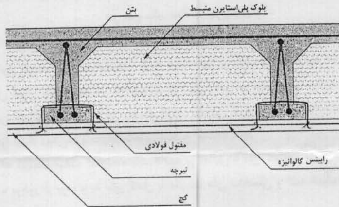
شکل ۱: یک نمونه جزئیات اجرایی قابل قبول برای اجرای اندود زیر بلوک سقفی پلی استایرن (حداکثر فواصل مفتولها برای اتصال رأبیتس به تیرچه، ۱۵ سانتی متر باشد)
